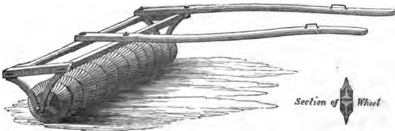
MILL ROLLER.
